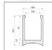
ПРОФИЛЬ ВЕРХНИЙ СТК-5
